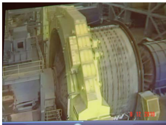
Molino de bola Minera “Pelambres”
